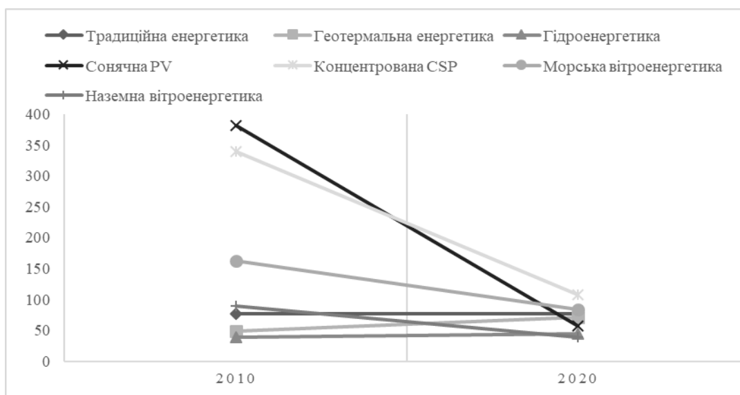
Рисунок 2 – Динаміка LCOE видів ВДЕ у світі ($ за МВт-год)
