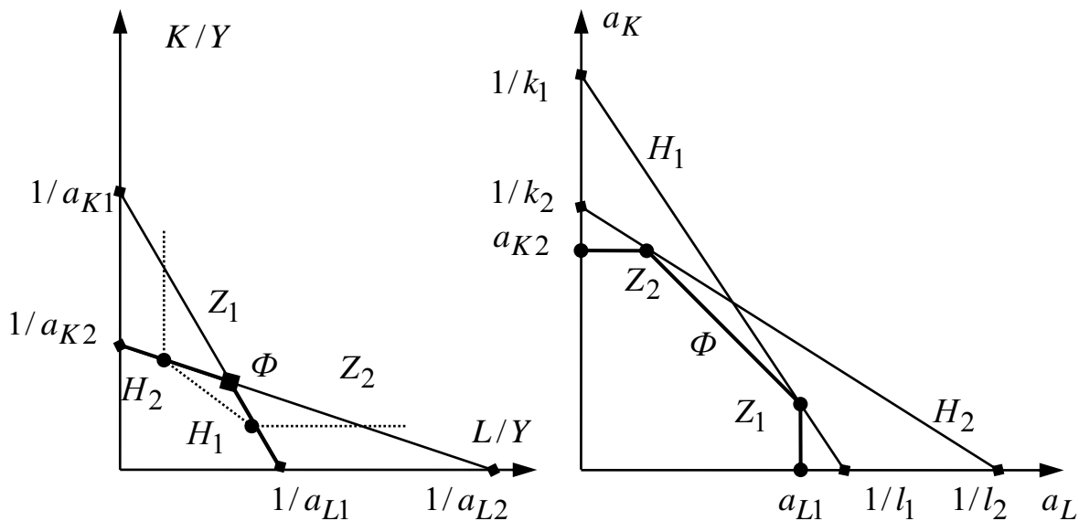
Рисунок 13 – СТР за методом оболонки фактичних виробничих функцій. Випадок ефективності лідерів
